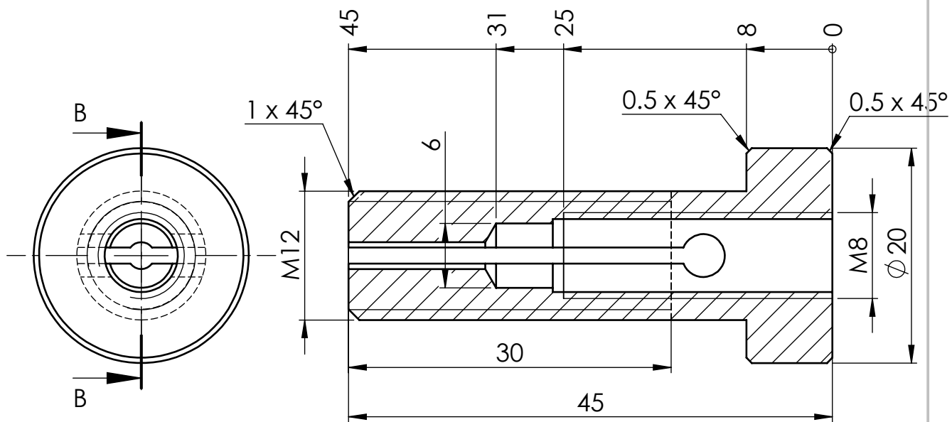
SEZIONE B-B
