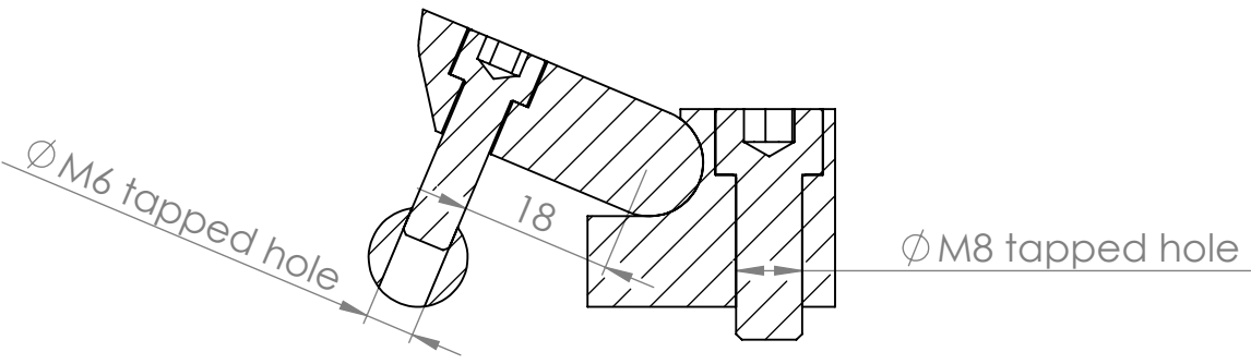
SECTION A-A
