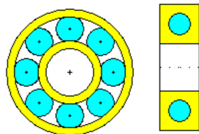
6201 12 x 32 x 10
