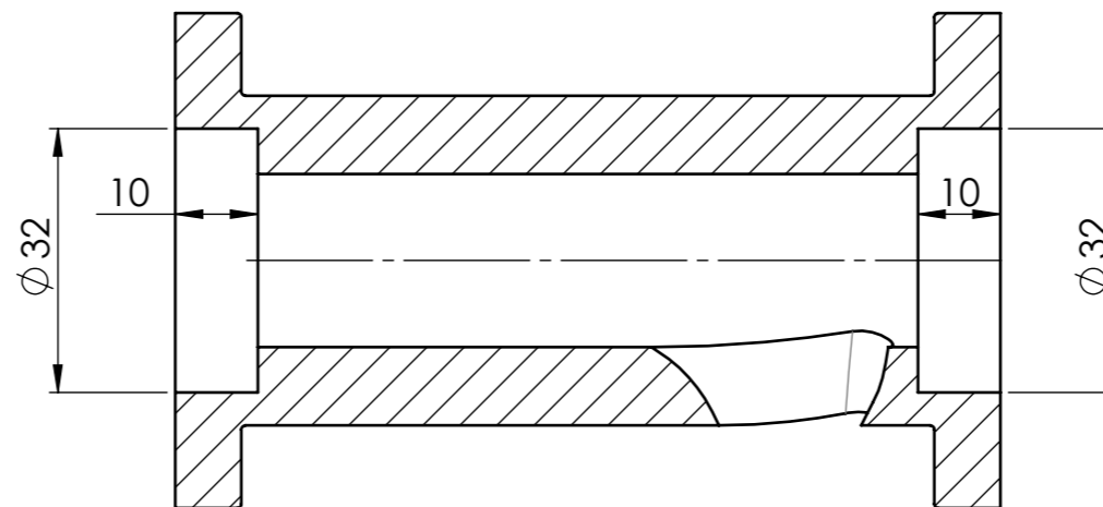
SEZIONE A-A
