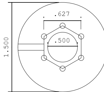
Right End 5/8 hex die
