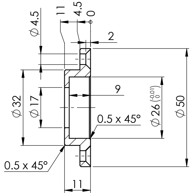
SEZIONE B-B
